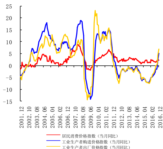
图 11 2001~2016 年江西省居民消费价格和生 产者价格变动趋势
