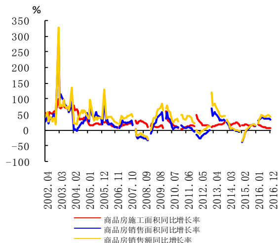
图 13 2002~2016 年江西省商品房施工和销售 变动趋势
