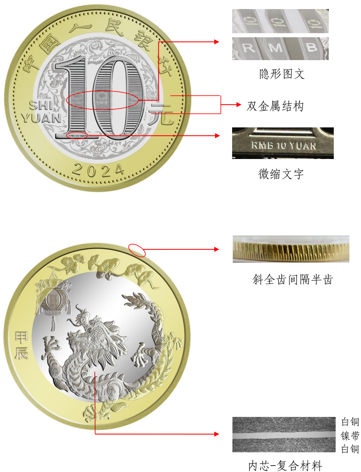
图 5 2024 年贺岁双色铜合金纪念币防伪特征示意图
